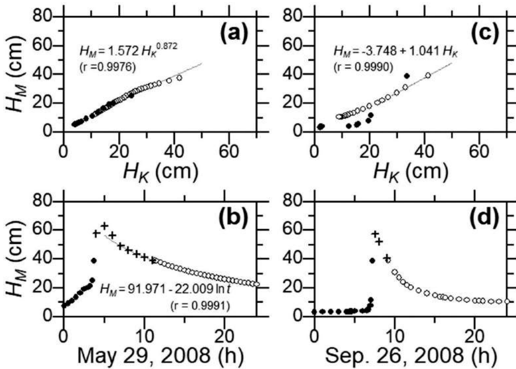
Fig. 4. 南谷における欠測期間（2008年5月29日（a, b）および同年9月26日（c, d））の推定水位 Estimated water stages during data missing periods (May 29 (a, b) and September 26 (c, d) in 2008). H_M : 南谷水位 water stages of the Minami-dani, H_K : 北谷水位 water stages of the Kita-dani, t : 欠測後の5月29日の時刻 time in hours after the data missing period on May 29 (b), ●: 欠測前の水位 water stages before data missing, ○: 欠測後の水位 water stages after data missing, +: 推定水位 estimated water stages.
