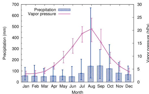
Fig. 2. 降水量および水蒸気圧の季節変化。 エラーバーは、対象期間内の最大・最小値。 Seasonal variations in precipitation and vapor pressure The error bars show the ranges for the observation period.
