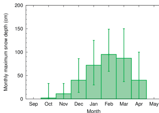
Fig. 3. 月最大積雪深の季節変化。 エラーバーは、対象期間内の最大・最小値。 Seasonal variation in monthly maximum snow depth The error bars show the ranges for the observation period.
